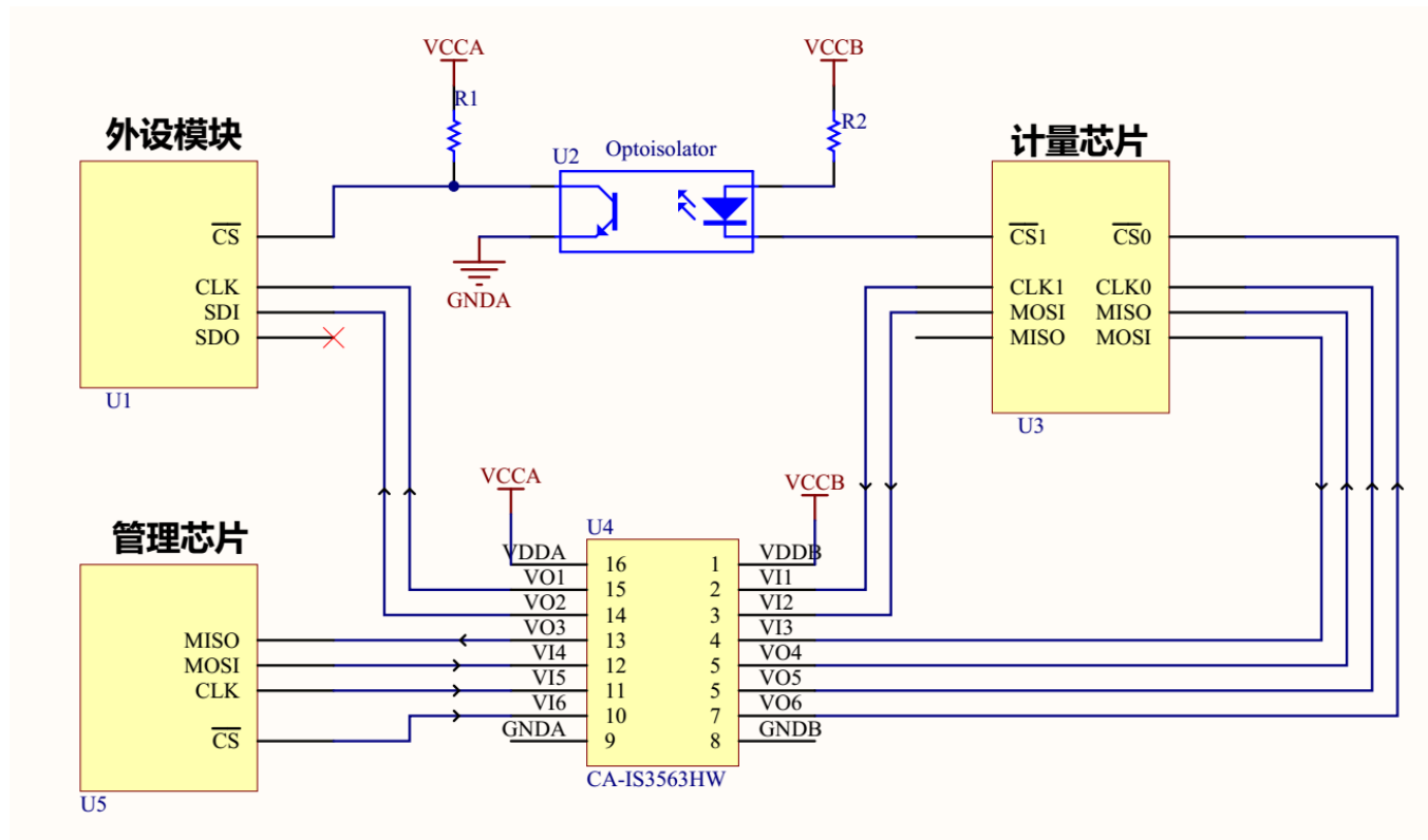
图 1-4 CA-IS3563 在三相双芯表中 SPI 通信接法示意图
