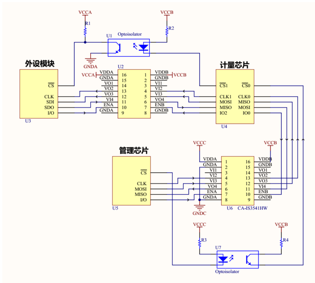
图 1-2CA-IS3541 在三相双芯表中 CS 用光耦 SPI 通信接法示意图
