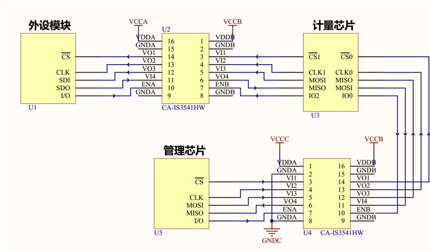
图 1-1 CA-IS3541 在三相双芯表中 SPI 通信接法示意图
