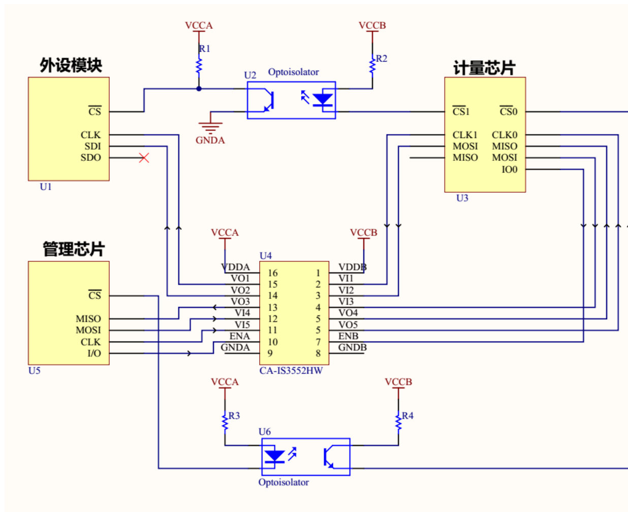
图 1-3 CA-IS3552 在三相双芯表中 SPI 通信接法示意图
