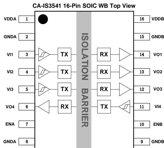
图 7-1 CA-IS3541 SOIC16-WB 宽体顶部视图
