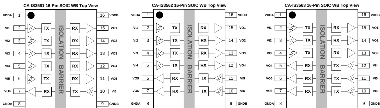
图 7-1 CA-IS356x 顶部视图
